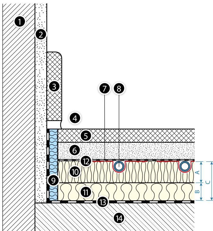
Pav. 30. Grindinis šildytuvas su System KAN-therm TBS plokštė ir papildoma izoliacija bei hidroizoliacija ant grindų perdangos, kontaktuojančių su gruntu
