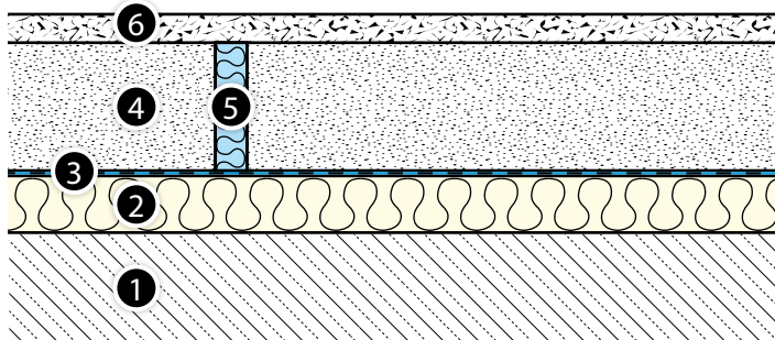
Pav. 14. Kompensacinės siūlės formavimas ant minkštos dangos.
