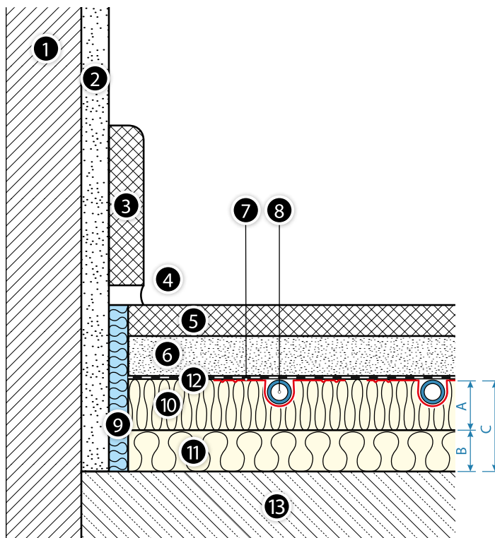
Pav. 29. Grindinis šildytuvas su System KAN-therm TBS plokštė ir papildoma izoliacija ant lubų perdangos virš nešildomos vidaus patalpos ir ant lubų perdangos, kontaktuojančių su išorės oru
