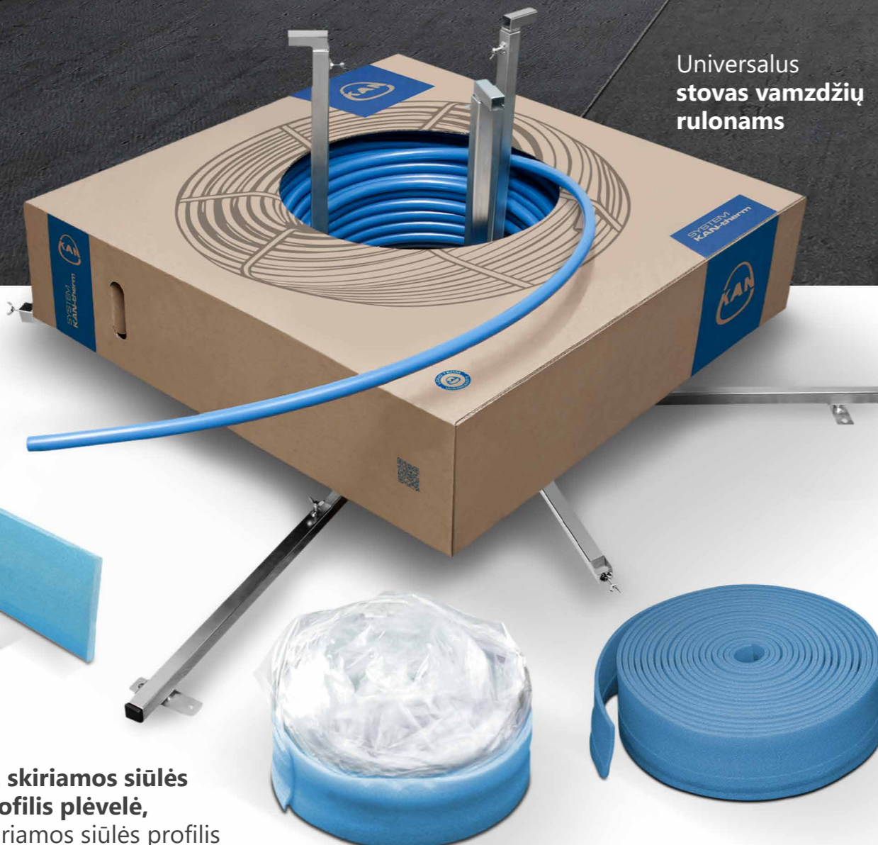
Pakraščių juosta su įpjovimu ir "sijonėliu"
